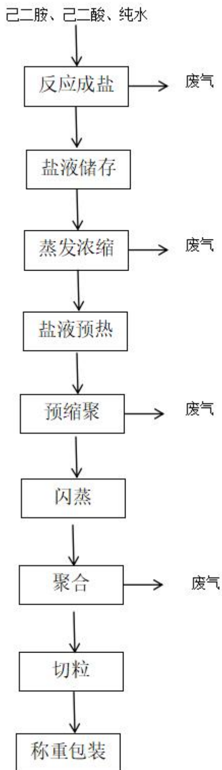
图 3-2 聚酰胺 66 生产工艺流程图
