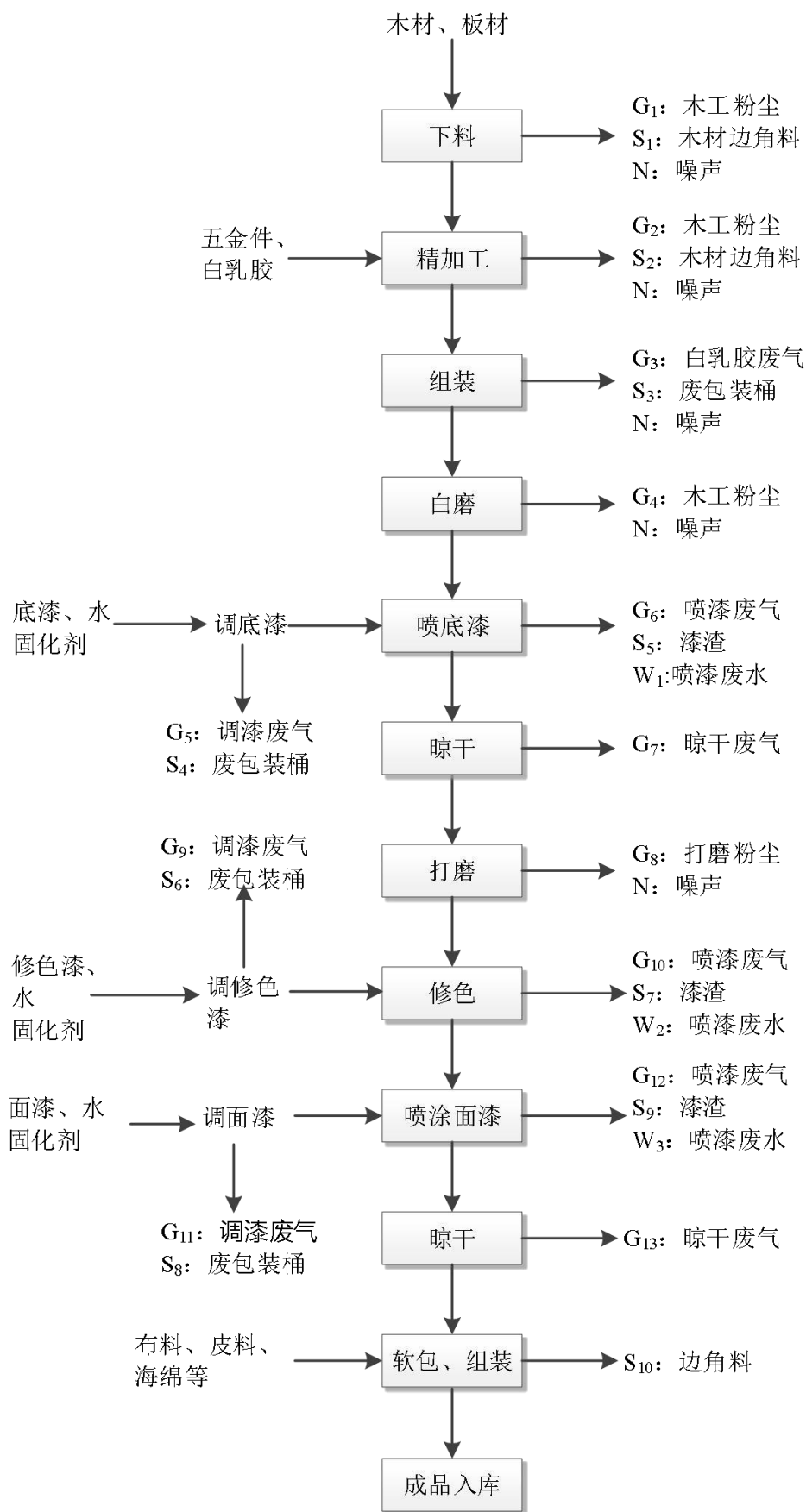
图1-3 生产工艺流程图
