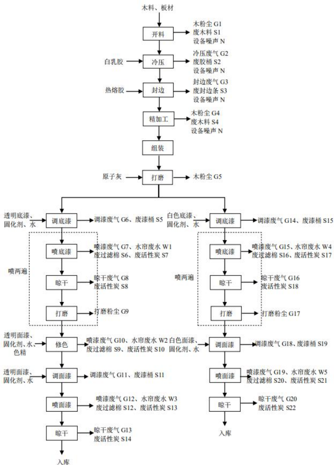
图 3-2 家具生产工艺流程及产污环节图
